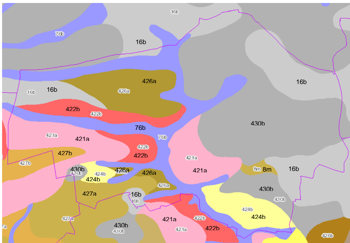
Abb. 30: Bodentypen im Gemeindegebiet Tuchenbach (Ausschnitt aus der Bodenübersichtskarte 1:25:000) 40
