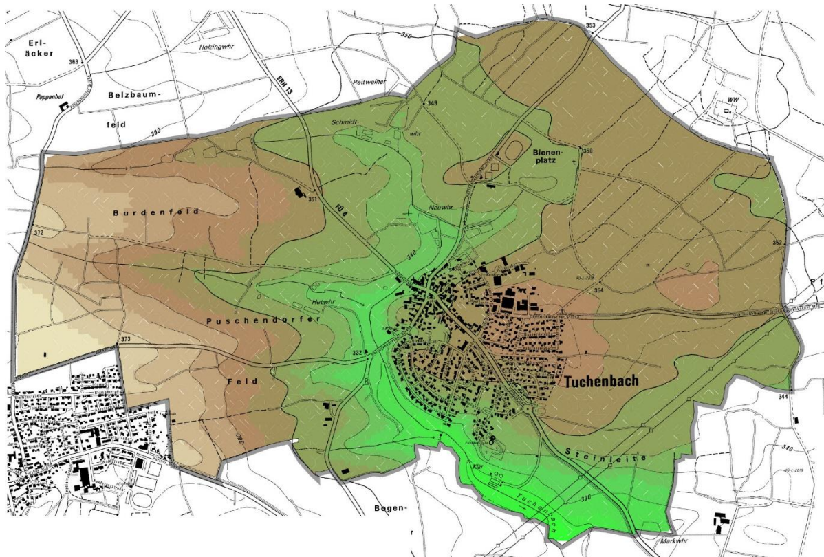
Abb. 6: Höhengschichtkarte 2
